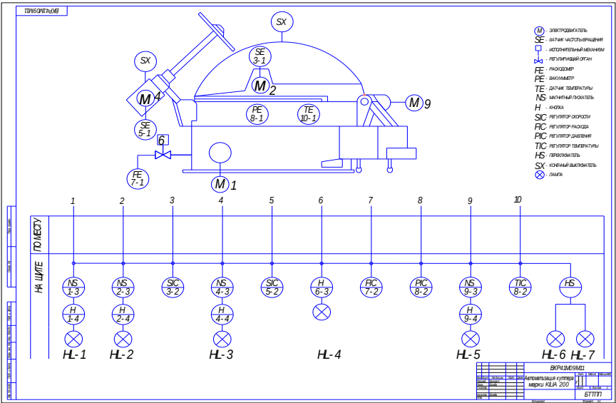
Рисунок 7 – Схема автоматизации куттера
